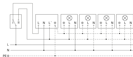
Schaltplan Anschluss über einen Wechselschalter für Dauerlicht- und Automatik-Betrieb
